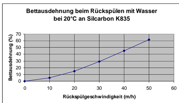
Abb. 1: Typische Betaausdehnungskurven für Aktivkohlen vom Typ K835
